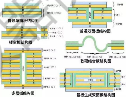
图2 柔性线路板的结构
