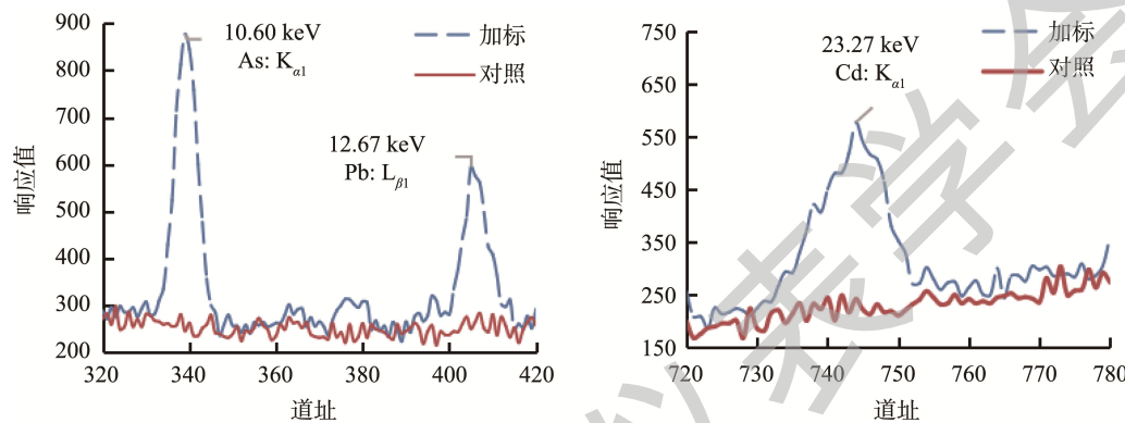
图 1 鲜香菇中 As、Pb、Cd 的 EDXRF 光谱
