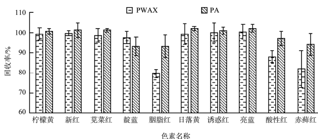
图 2 PA 与 PWAX 固相萃取柱对 10 种合成色素的回收率( n=3 )
