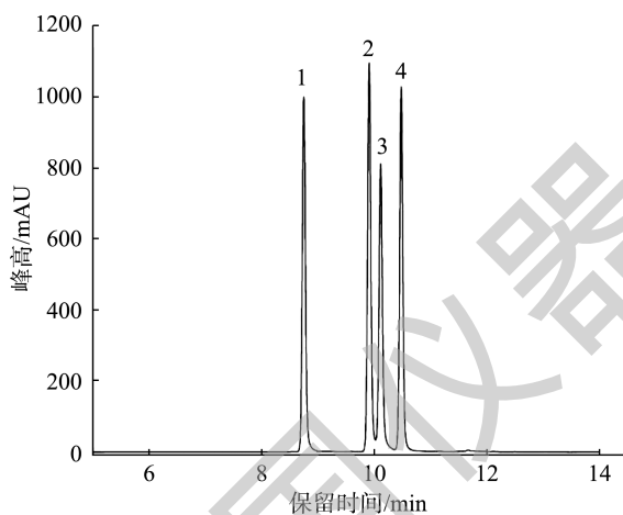
图1 4种待测物的色谱峰
